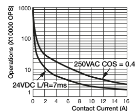
fig. 3. Gleichstrom-Grenzlastkurve
