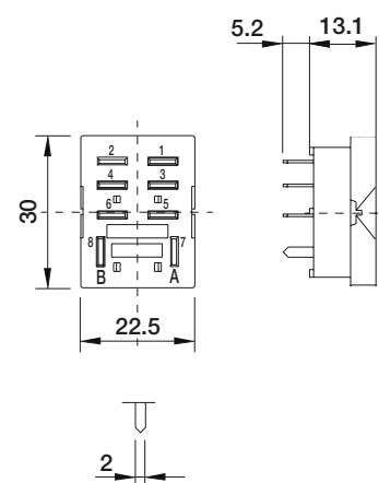
fig. 2. Abmessungen (mm)
