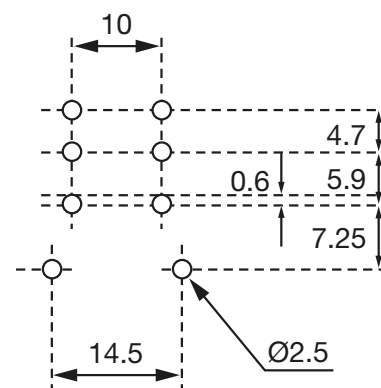
fig. 2. Abmessungen (mm)
