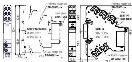
fig. 4. Dimensions (mm)
