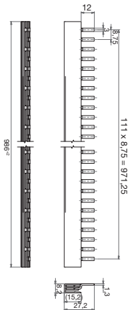
fig. 1. Abmessungen (mm)
