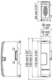
fig. 1. Dimensions (mm)
