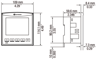
fig. 1. Dimensions (mm)
