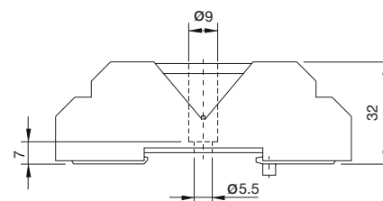
fig. 2. Abmessungen (mm)
