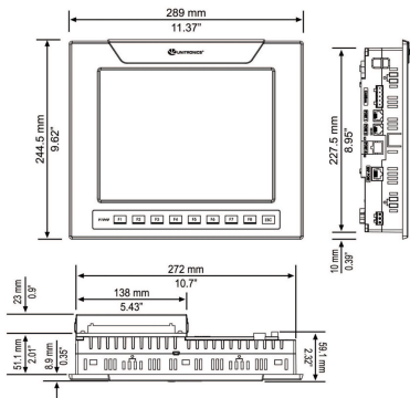
fig. 1. Dimensions (mm)
