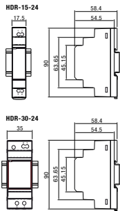
fig. 1. Abmessungen (mm)
