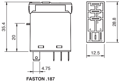
fig. 4. Dimensions (mm)
