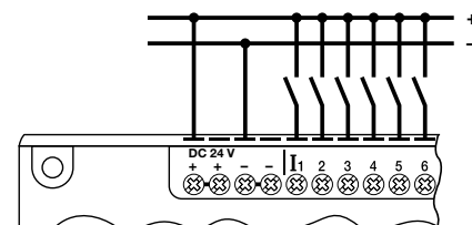
fig. 1. Wiring diagram
