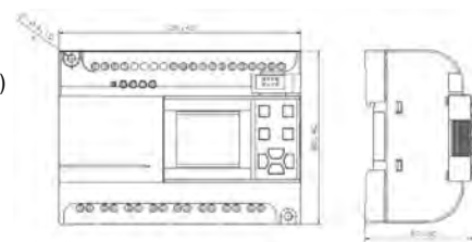
fig. 2. Abmessung (mm)
