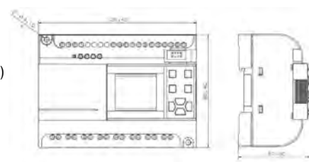
fig. 2. Abmessung (mm)
