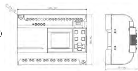
fig. 2. Abmessung (mm)
