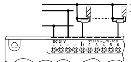
fig. 1. Wiring diagram
