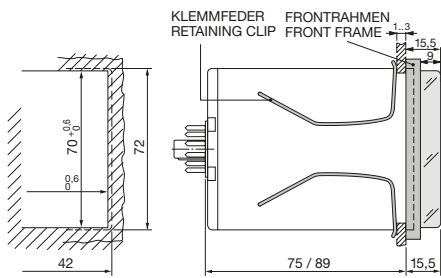
fig. 1. Abmessungen (mm)
