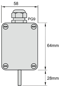
fig. 1. Dimensions (mm)
