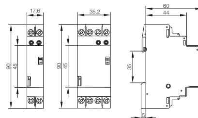
fig. 3. Dimensions (mm)
