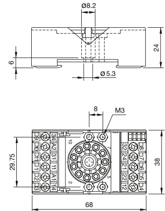
fig. 2. Abmessungen (mm)
