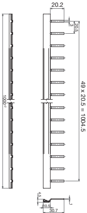
fig. 1. Dimensions (mm)
