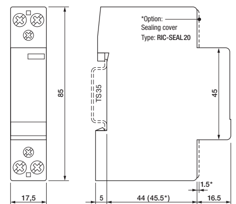
fig. 3. Abmessungen (mm)
