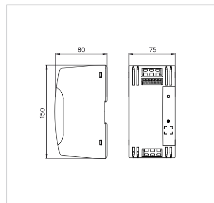
«Plan coté e» 75 mm Module
