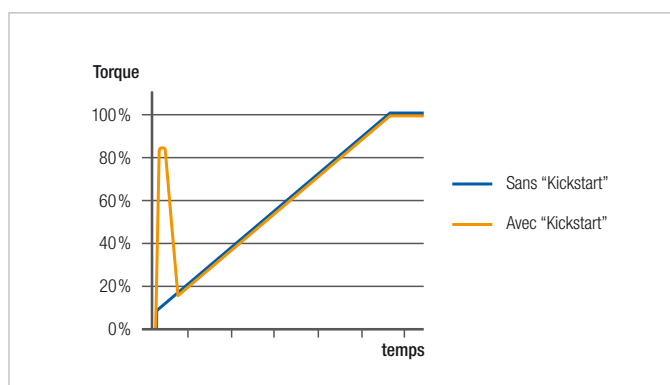
Réglage du couple de démarrage avec CCM
