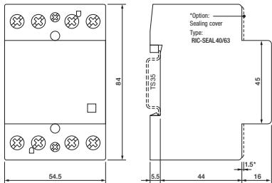
fig. 3. Dimensions (mm)
