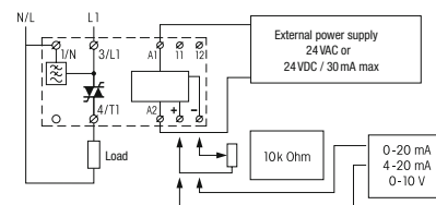
fig. 1. Wiring diagram
