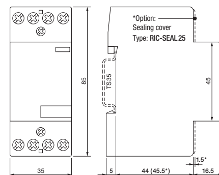
fig. 3. Abmessungen (mm)
