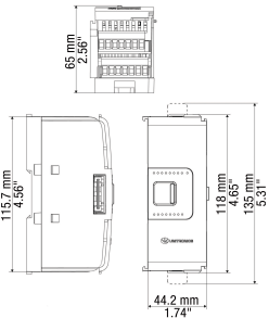
fig. 1. Abmessungen (mm)
