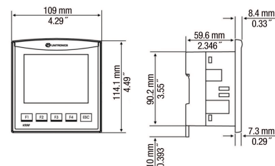
fig. 1. Abmessungen (mm)
