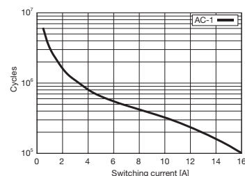
fig. 2. Wechselstrom-Schaltzyklen
