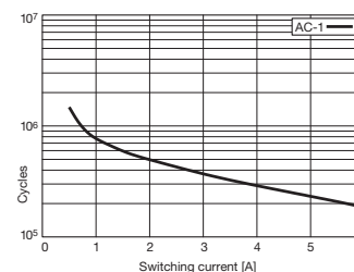
fig. 3. Gleichstrom-Grenzlastkurve
