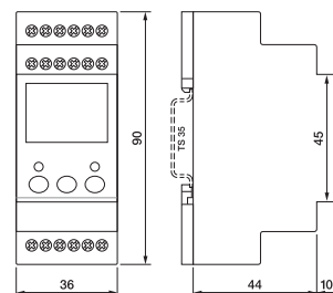
fig. 4. Abmessungen (mm)
