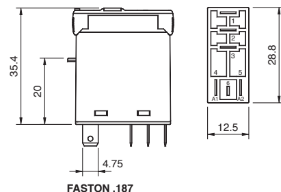
fig. 4. Dimensions (mm)
