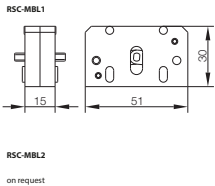
fig. 1. Abmessungen (mm)
