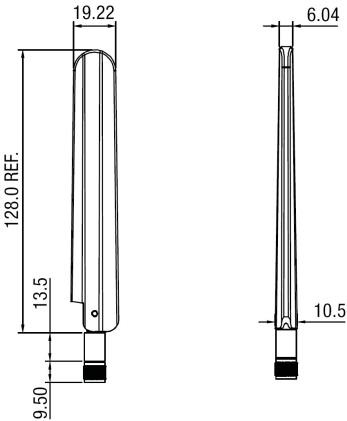
fig. 1. Abmessungen (mm)
