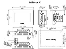
fig. 1. Dimensions (mm)
