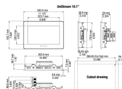
fig. 1. Abmessungen (mm)
