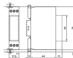
fig. 4. Abmessungen (mm)
