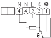
fig. 1. Wiring diagram
