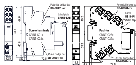
fig. 1. Abmessungen (mm)
