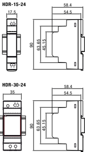
fig. 1. Dimensions (mm)
