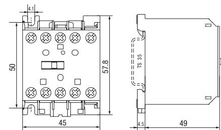
fig. 3. Dimensions (mm)
