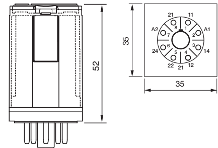
fig. 4. Dimensions (mm)
