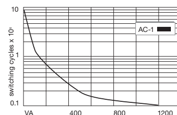
fig. 3. Gleichstrom-Grenzlastkurve
