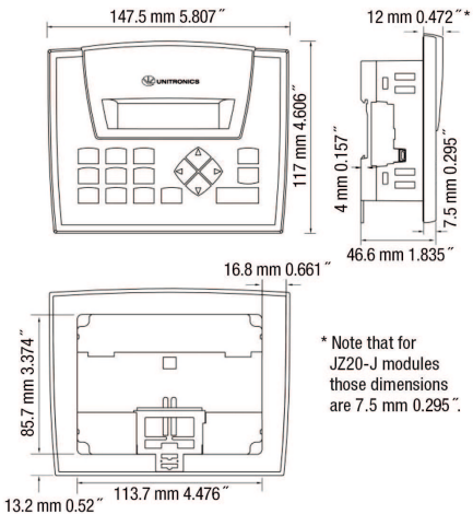
fig. 1. Dimensions (mm)
