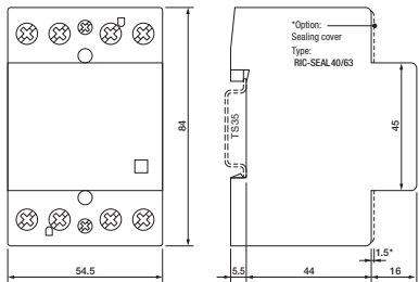
fig. 3. Dimensions (mm)
