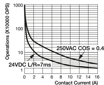
fig. 3. Gleichstrom-Grenzlastkurve
