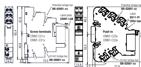
fig. 4. Abmessungen (mm)
