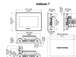
fig. 1. Abmessungen (mm)
