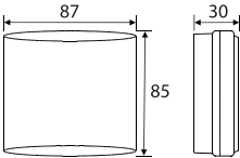
fig. 2. Abmessungen (mm)
