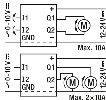
fig. 2. Funktionsdiagramm
