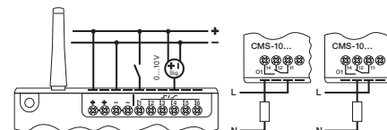
fig. 2. Max. Ausschaltvermögen RZ
