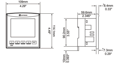
fig. 1. Abmessungen (mm)
