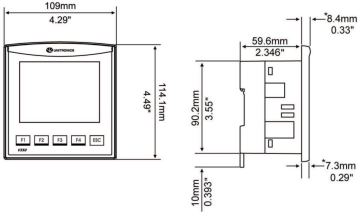
fig. 1. Dimensions (mm)
