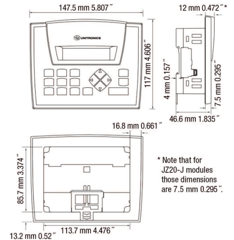
fig. 1. Dimensions (mm)
