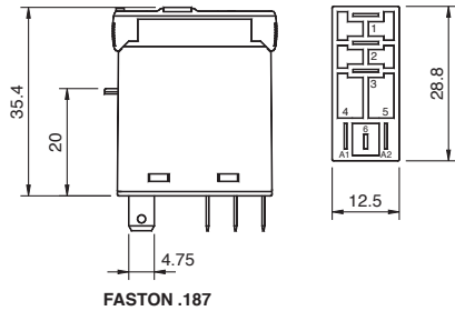
fig. 4. Dimensions (mm)
