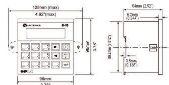
fig. 1. Dimensions (mm)
