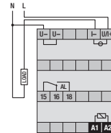
fig. 2. Wechselstrom-Schaltzyklen
